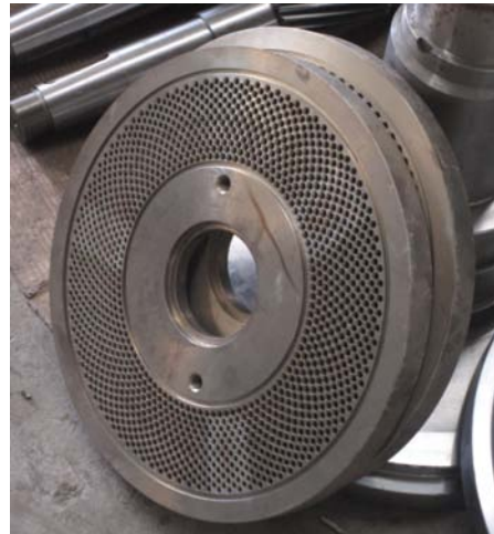
Flat die for big flat die pellet mill
